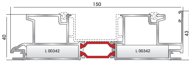
15010 W=2662gr/m A=0,636m 2 /m Double track
