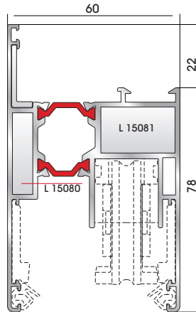
15025 W=1945gr/m A=0,598m 2 /m Window/balcony door sash
